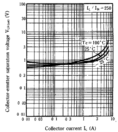
V_{CE(sat)} - I_C
