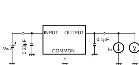
Fig.1 出力電圧、入力安定度、負荷安定度、出力電圧温度係数測定回路
