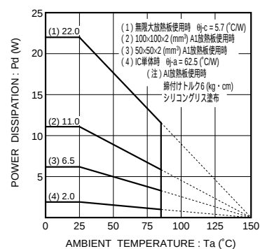
Fig.9 熱軽減特性 (TO220)
