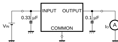
Fig.4 最小入力電圧差測定回路
