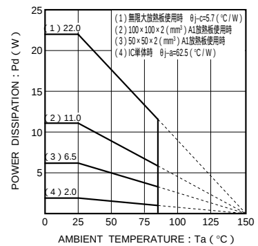
Fig.9 熱軽減特性 (TO220FP)
