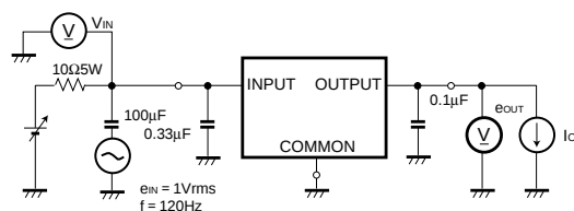
Fig.2 リップルリジェクション測定回路
