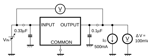
Fig.4 最小入力電圧差測定回路
