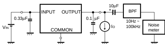
Fig.3 出力雑音電圧測定回路
