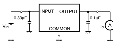
Fig.4 最小入力電圧差測定回路
