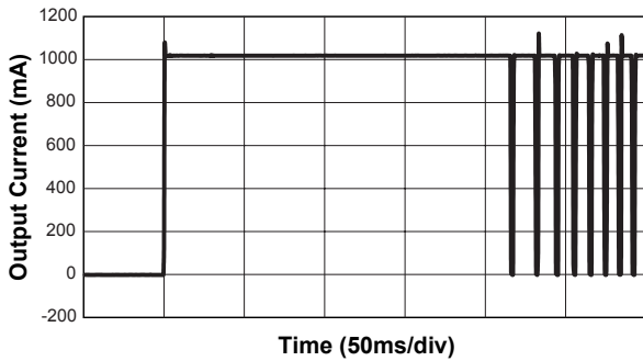
LDO Over-Current Protection (EN = GND; ENLDO = V_{IN} )
