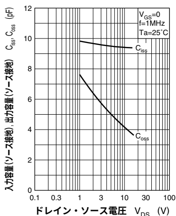
C_{iss}, C_{oss} - V_{DS}
