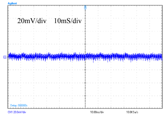
Vin=265V, Io=1A
