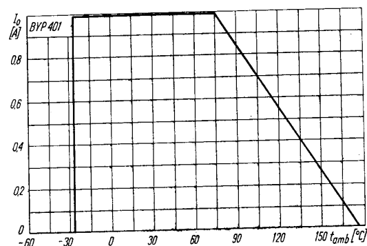
Dopuszczalny prąd wyprostowany w funkcji temperatury otoczenia I_O = f(t_{amb})
