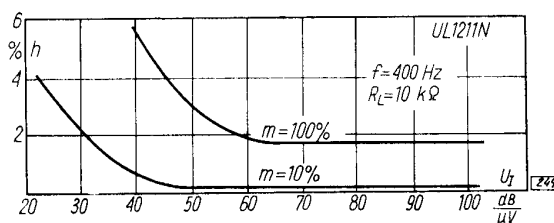
Współczynnik zawartości harmoniczných w funkcji napięcia wejściowego dla toru FM
