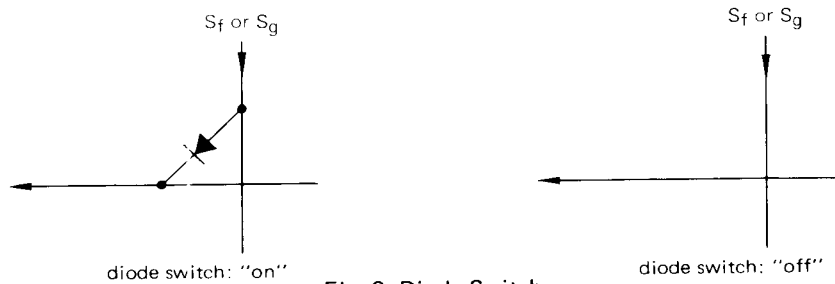
Fig. 3 Diode Switch
