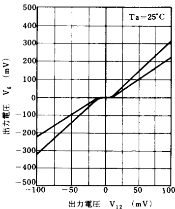
色差クリップ回路入出力特性
