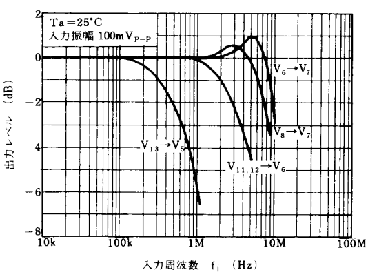
周波数特性
