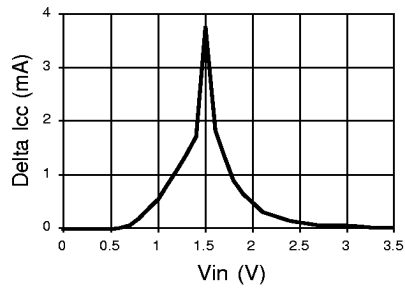
Delta Icc vs Vin (1 input)
