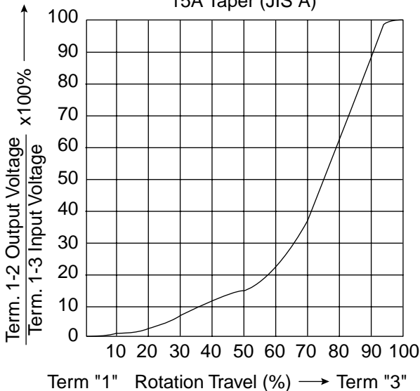
15A Taper (JIS A)
