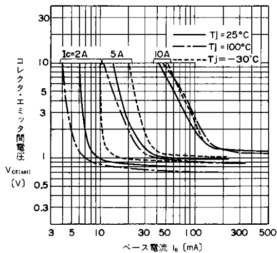
出力特性
