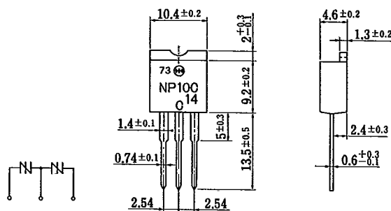
外形図 Outline Dimensions
