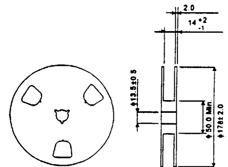
178 mm/7" Reel
