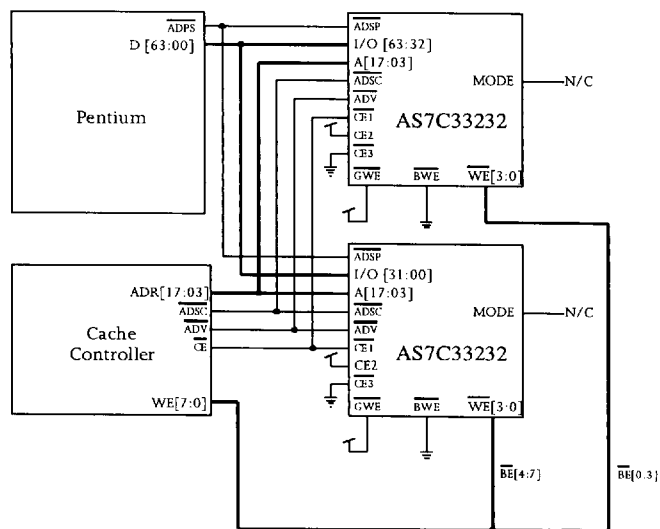
Figure A: Pentium 256KB cache
