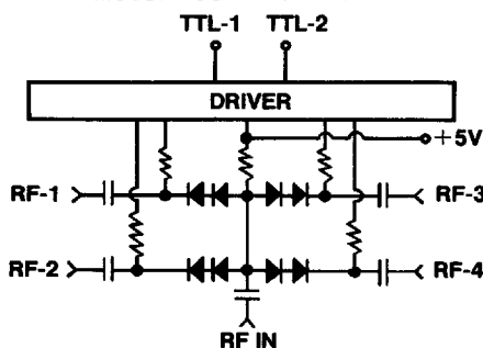
TTL LOGIC FOR ZSDR-425 & TOSW-425
