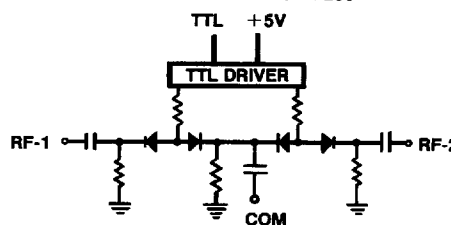
TTL LOGIC FOR ZSDR-230 & TOSW-230
