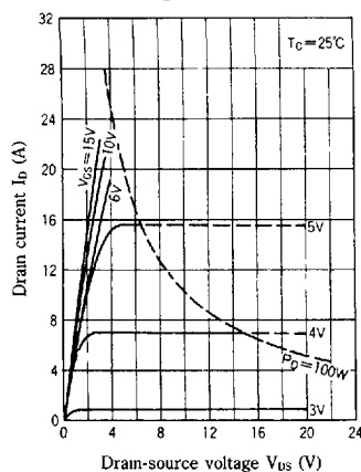
I_D - V_{DS}
