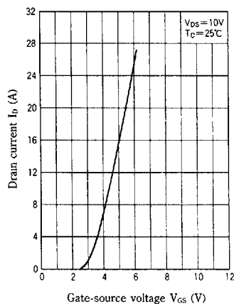
I_D - V_{GS}
