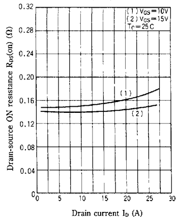
R_{DS(on)} - I_D
