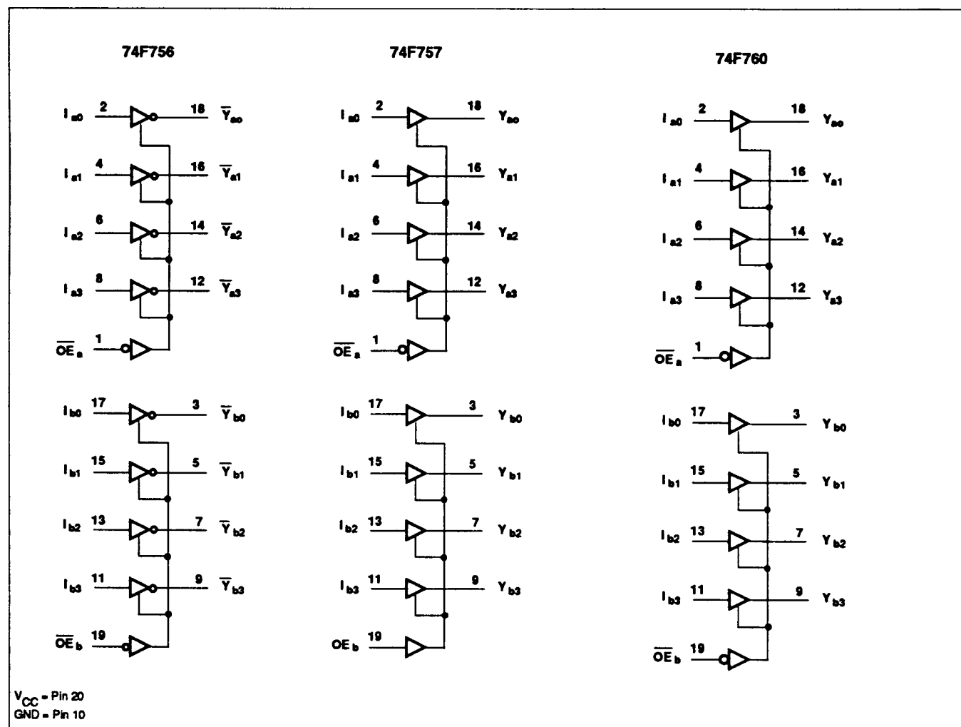
FUNCTION TABLE, 74F756
