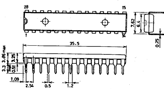
Package Dimensions 3133 (unit : mm)
