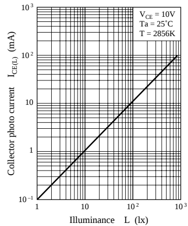
I_{CE(L)} - L
