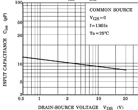
C_{iss} - V_{DS}
