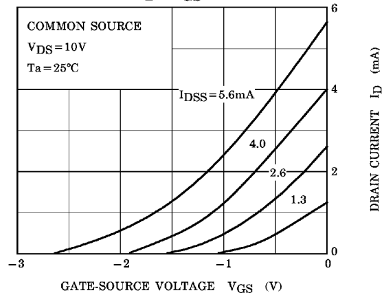
I_D - V_{GS}
