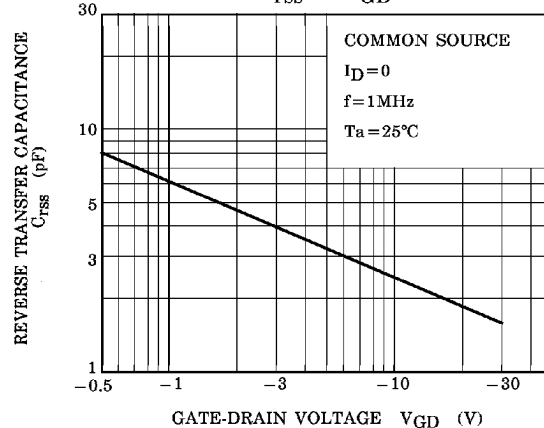
C_{rss} - V_{GD}
