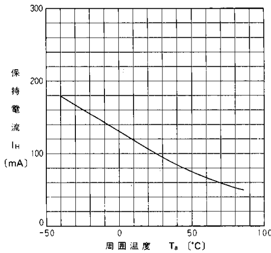
保持電流—温度依存性(代表特性) Dynamic Holding Current
