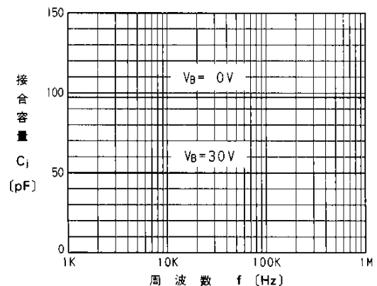
接合容量—周波数依存性(代表特性) Junction Capacitance
