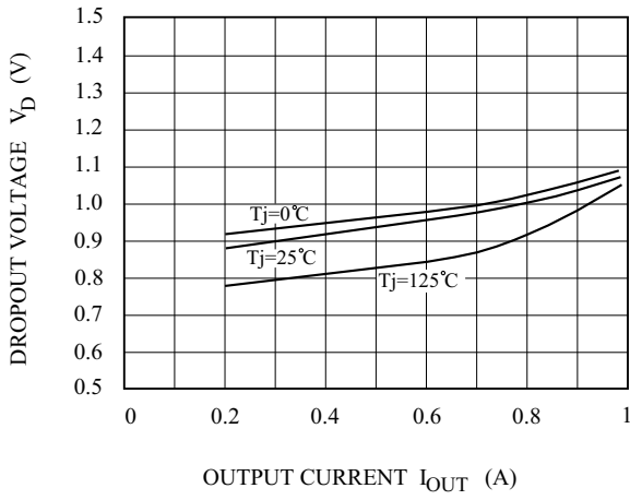
Fig. 3 V_D - I_{OUT}
