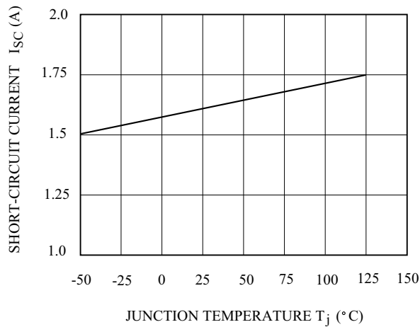
Fig. 7 I_{SC} - T_j
