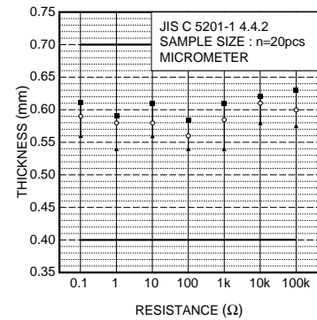
Fig.4 寸法 (厚さ)
