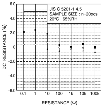
Fig.5 抵抗値
