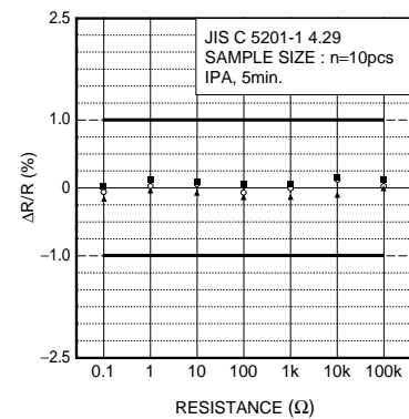
Fig.13 耐溶剤性
