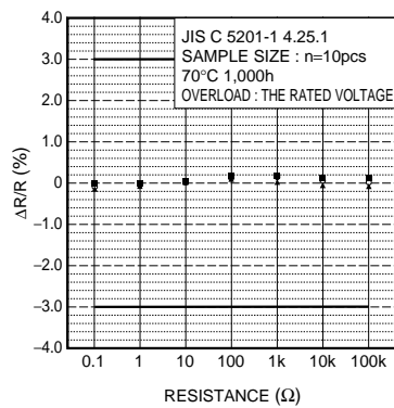
Fig.11 70°Cでの耐久性
