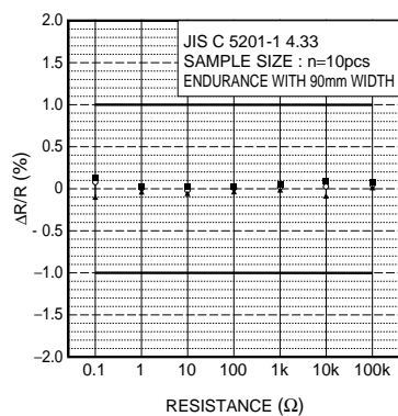
Fig.14 耐プリント板曲げ性
