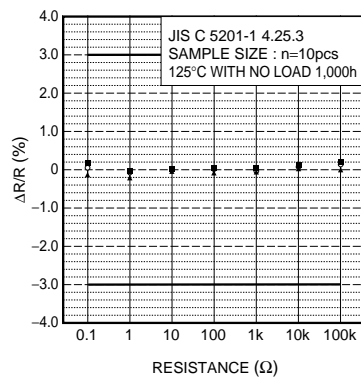
Fig.12 耐久性
