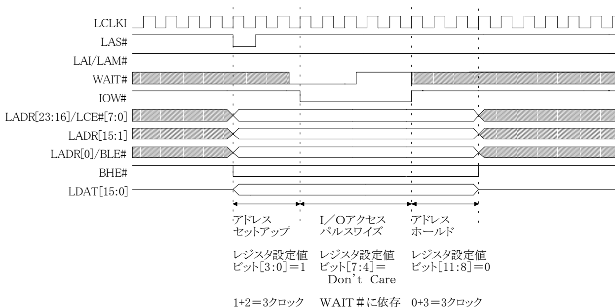
図22. I/Oライトアクセス(WAIT#使用)
