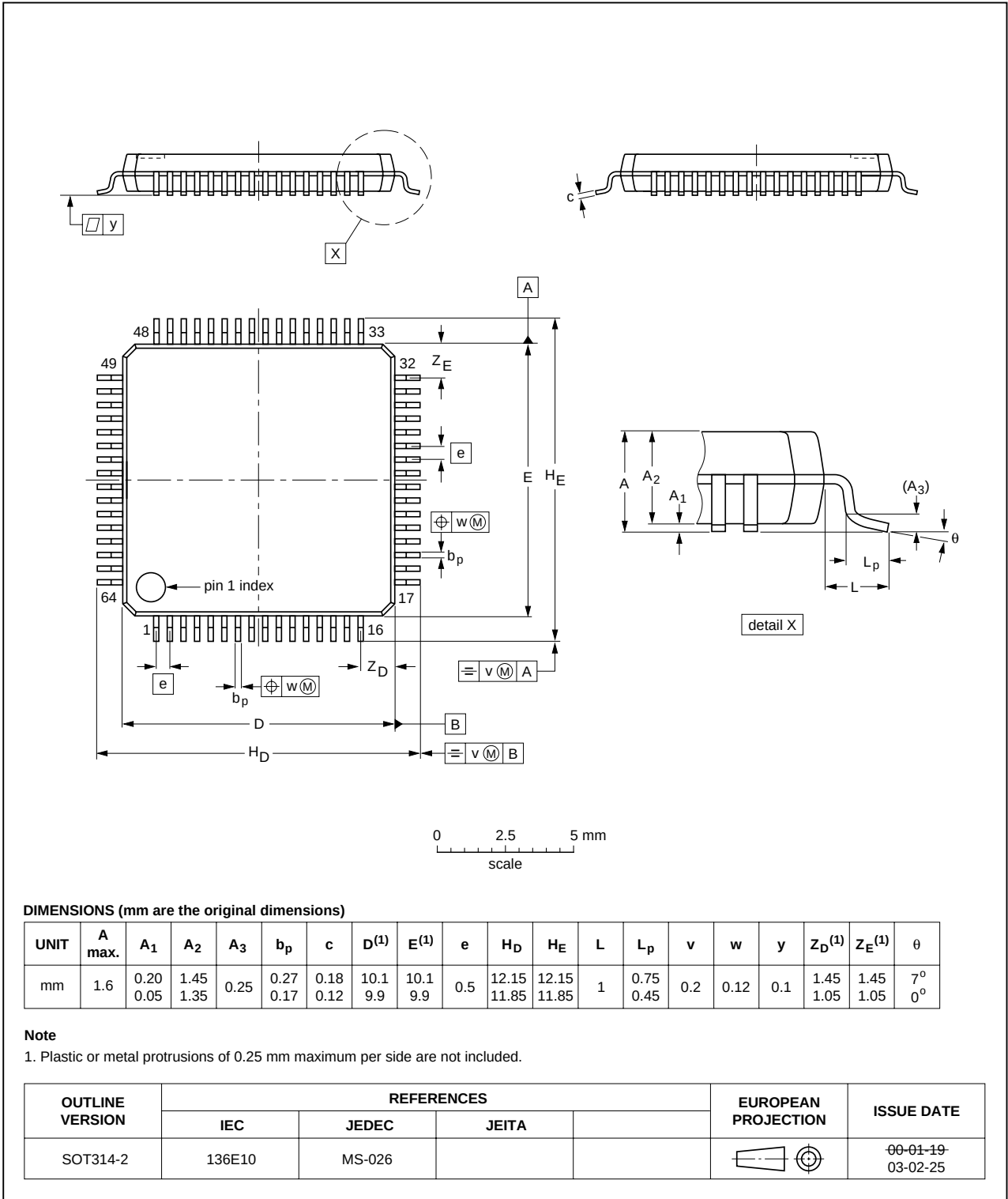
Fig 6. SOT314-2 (LQFP64).
