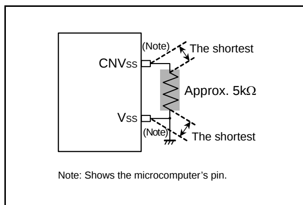
Fig. 113 Wiring for the CNVss
