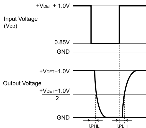
CMOS Output
