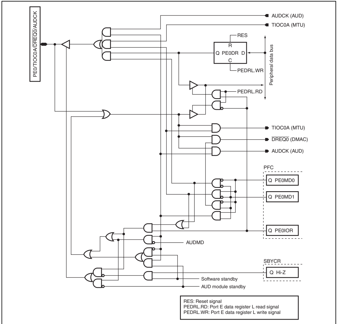
Figure D.46 PE0/TIOC0A/DREQ0/AUDCK
