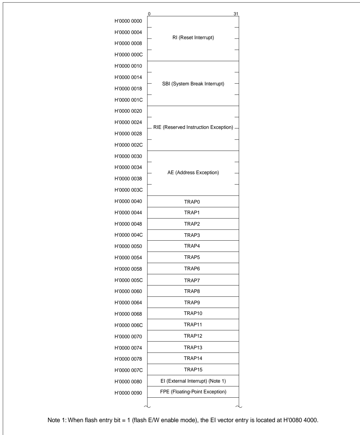
Figure 3.5.1 EIT Vector Entry
