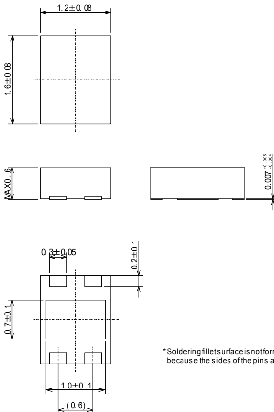
USP-4
