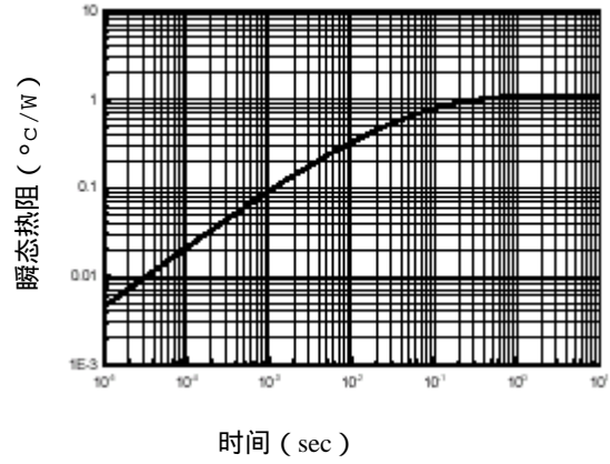
图四、热响应
