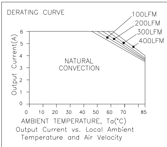
V_o=0.75\text{ V}
