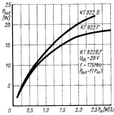
Bild 11: Ausgangsleistung als Funktion der Eingangsleistung beim KT 922 B und KT 922 Г
