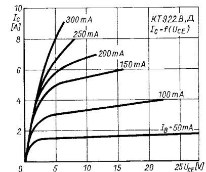
Bild 9: Ausgangskennlinienfeld der Typen KT 922 B und KT 922 Д
