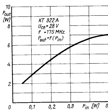
Bild 10: Ausgangsleistung als Funktion der Eingangsleistung beim KT 922 A
