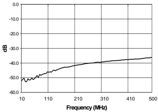
L-I Isolation
