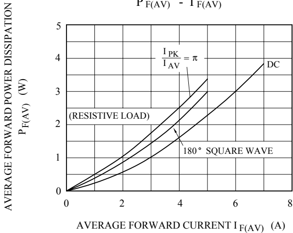
P_{F(AV)} - I_{F(AV)}
