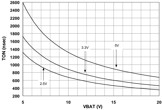
TON vs. VBAT - VOUT ≥ 2.5V
