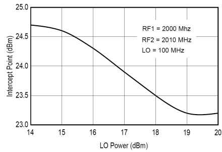
IIP3 vs. LO Power
