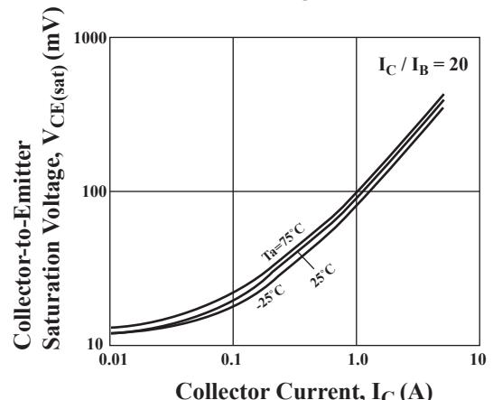
FIG.4 V_{CE(sat)} - I_C
