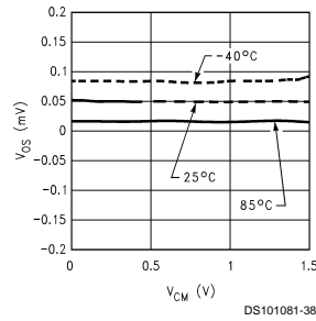
V_{OS} vs. V_{CM} V^+ = 2.7V
