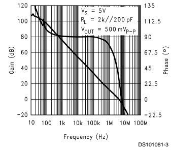
Gain/Phase
