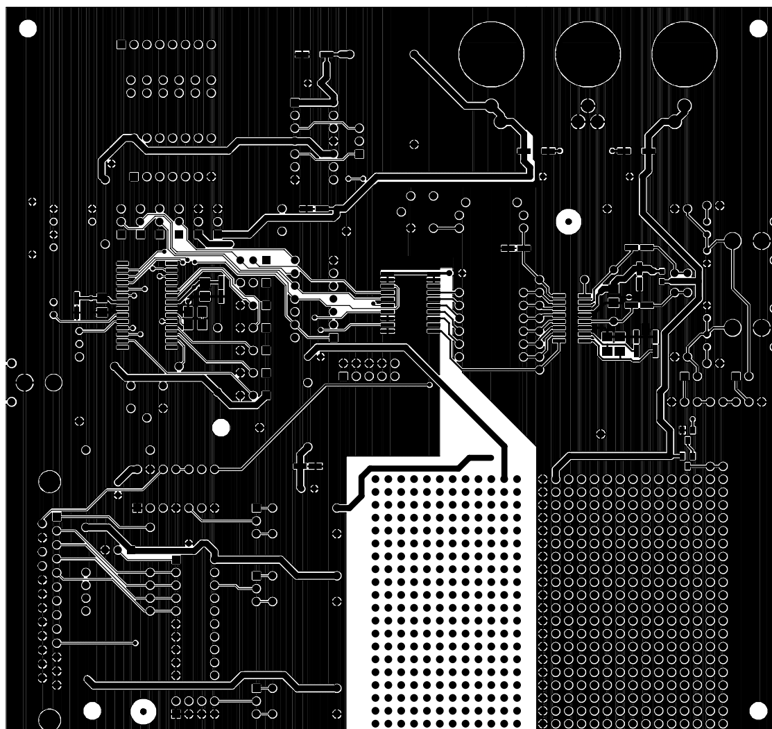
TOP SIDE
