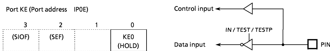
Figure 3-9. Port KE
