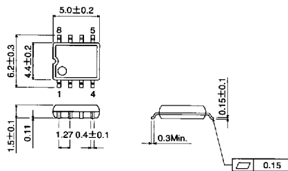
SOP8
