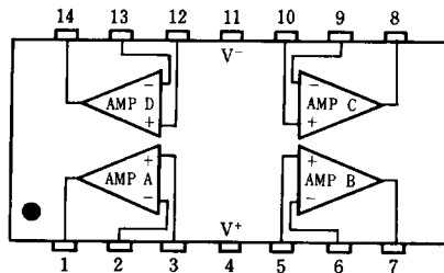
NJM2138M NJM2138V
