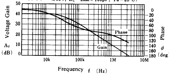
NJM072B/082B
