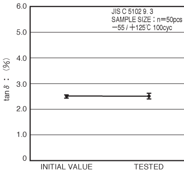
Fig.11 \tan \delta
