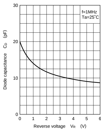
C_t - V_R
