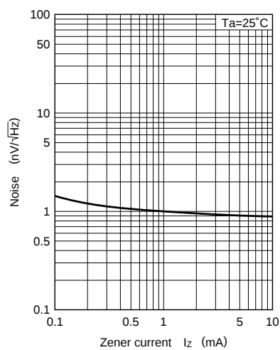
Noise - I_Z
