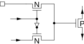
Fig. 3–12: Input pin 61
