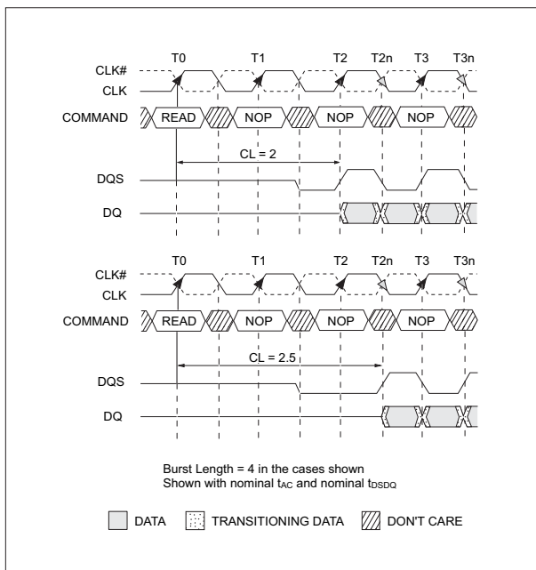
FIG. 4 CAS LATENCY
